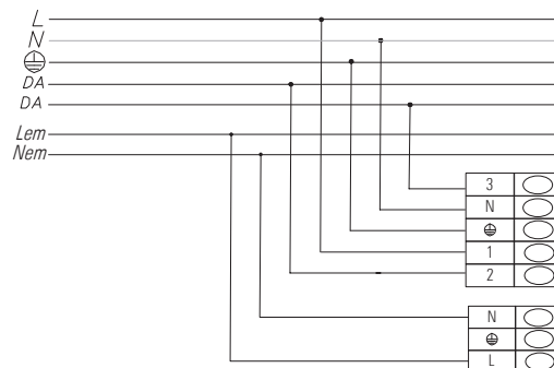
11-DALI EM (5+3 core cable) 5P+3P
