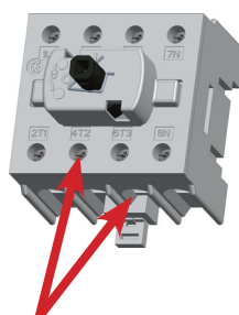
PZ2 2,5 Nm 2,5-35 mm 2 Cu *
