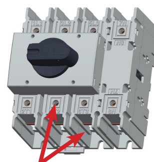
HEX 4mm 6 Nm 6-70 mm 2 Cu
