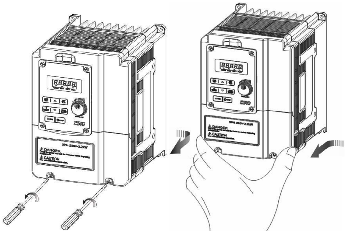
Etape 1 : Devisser les vis
