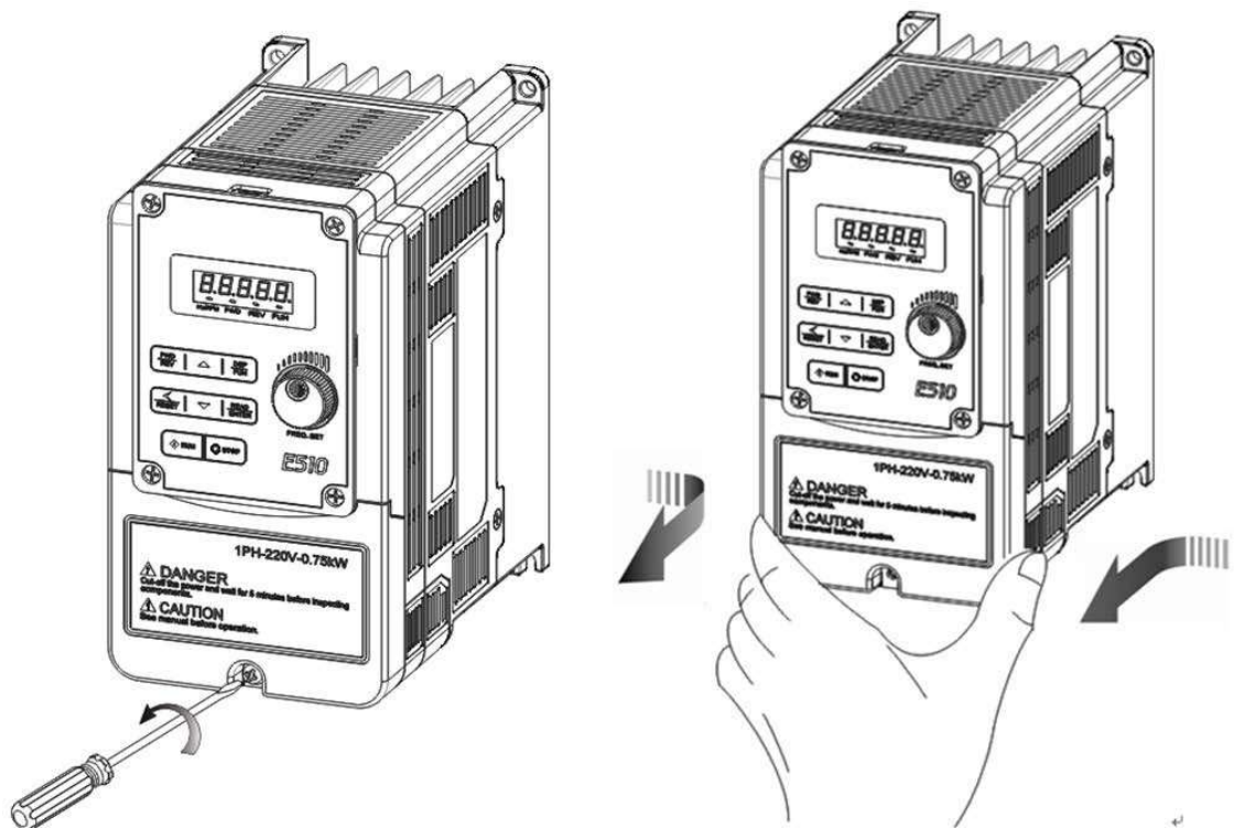
Etape 1 : Devisser la vis
