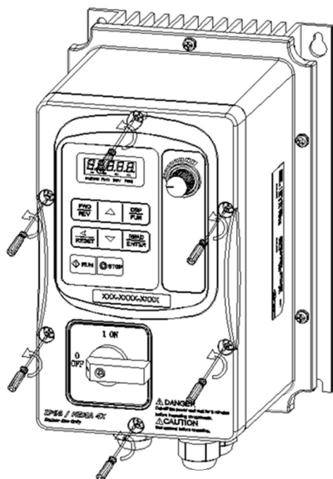
Etape 1 : Devisser les vis
