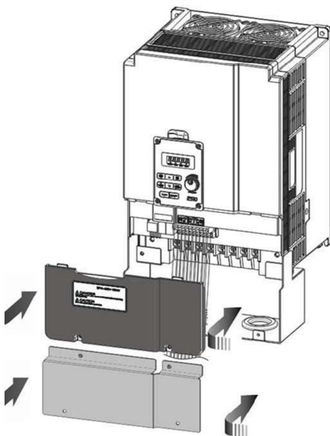
Etape 3 : Remettre les caches
