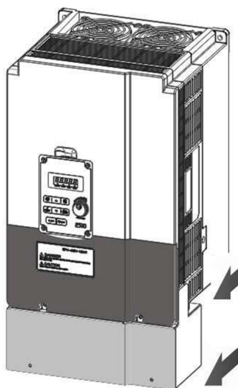
Etape 2 : Retirer les caches
