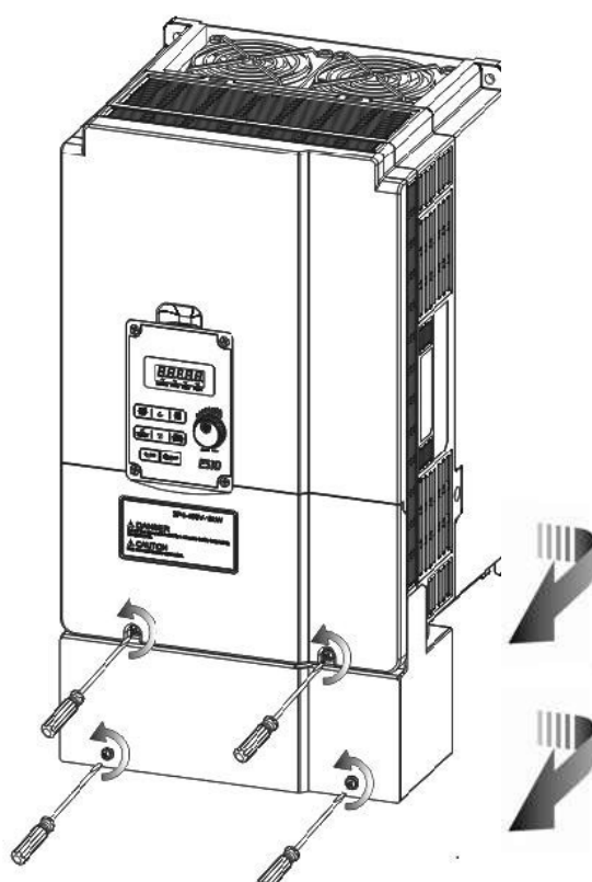
Etape 1 : Devisser les vis
