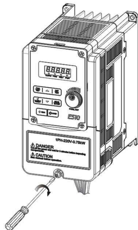
Etape 4 : Revisser la vis
