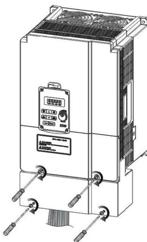
Etape 4 : Revisser les vis
