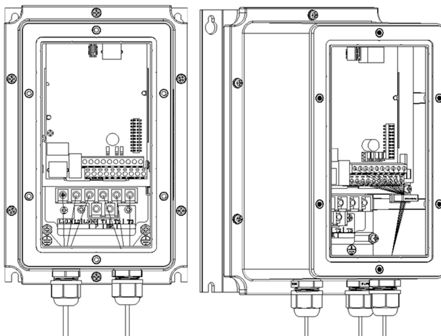
Etape 5 : Brancher les cables d'alimentation et les cables moteur en passant à travers les presse-étoupes
