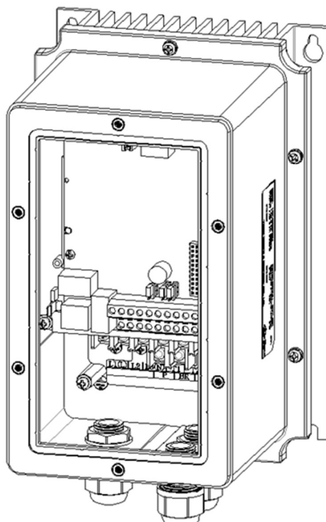
Etape 4 : utiliser les presse-étoupes étanches prévus pour connecter les câbles
