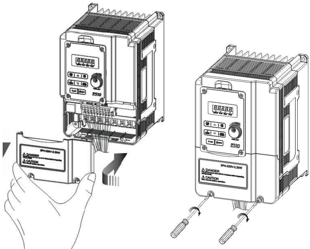
Etape 3 : Remettre le cache
