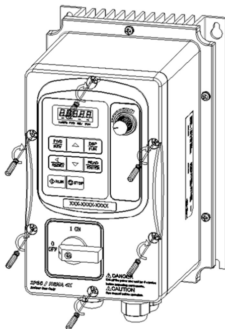
Etape 7 : Vérifier le serrage des presse-étoupes et s'assurer que la face avant est bien en place. Resserer les vis.
