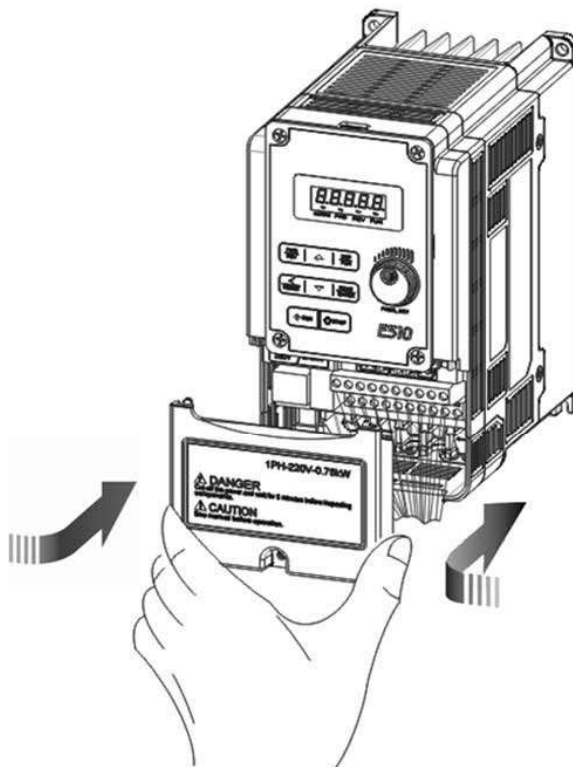
Etape 3 : Remettre le cache
